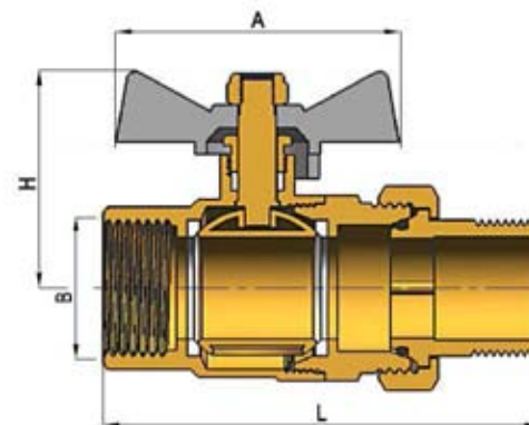
Рис 2. Основные габаритные размеры
