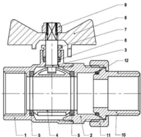
Рис 1. Основные элементы конструкции
