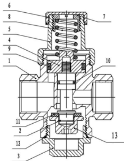
Рис 1. Основные элементы конструкции
